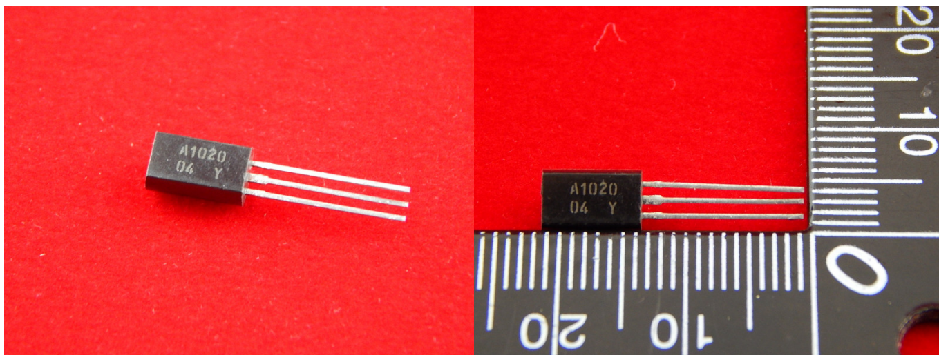
2SA1020, Транзистор PNP 50B 2A [TO92MOD]
