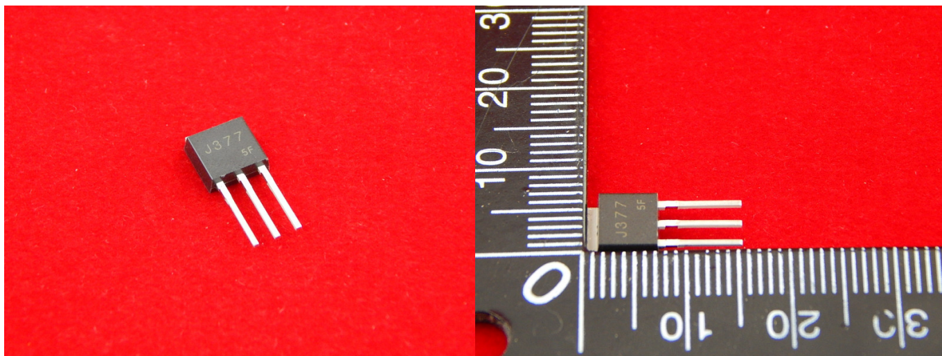
Транзистор 2SJ377, MOSFET
