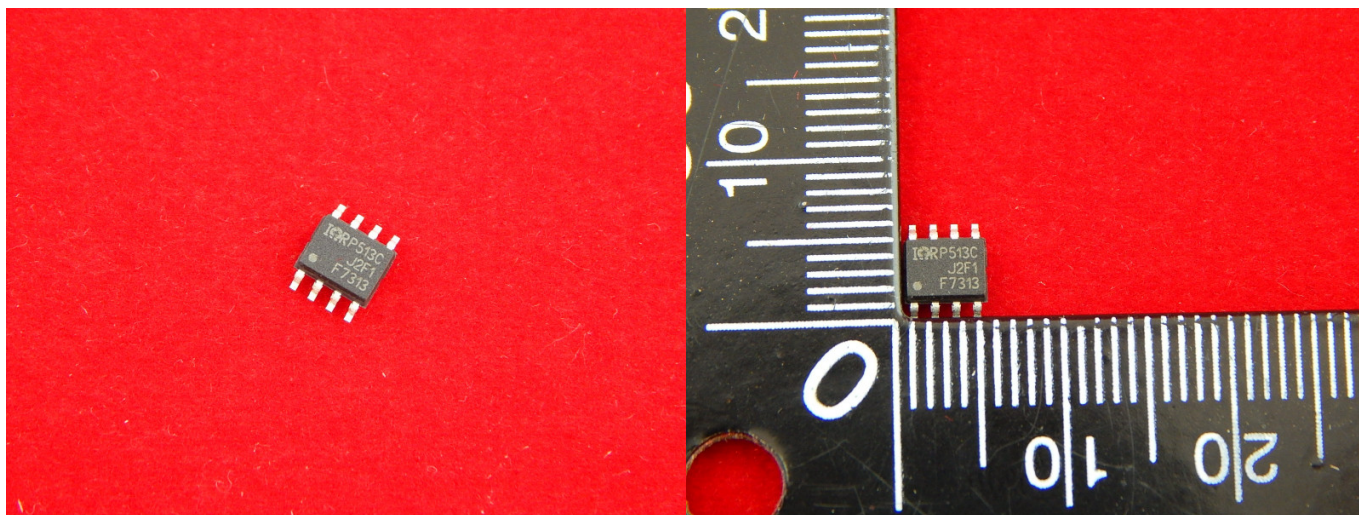
Полевой транзистор IRF7313PBF, 2N-канала 30В 6.5А в корпусе SO8
