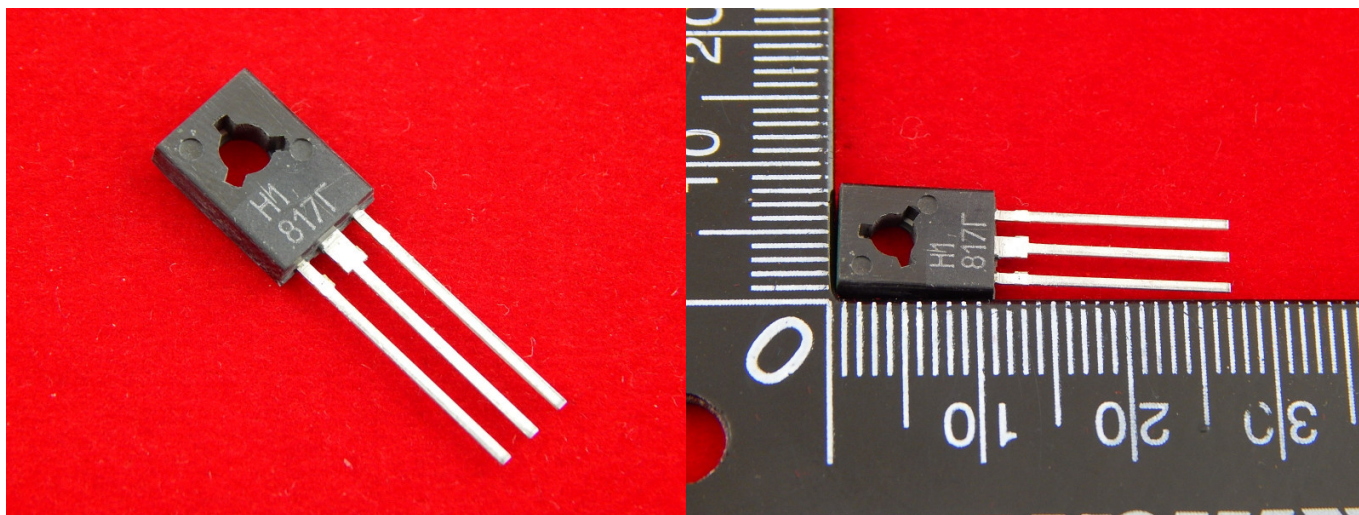
КТ817Г (BD237), Транзистор NPN 100В 3А 25Вт 3МГц ТО126 (КТ-27)
