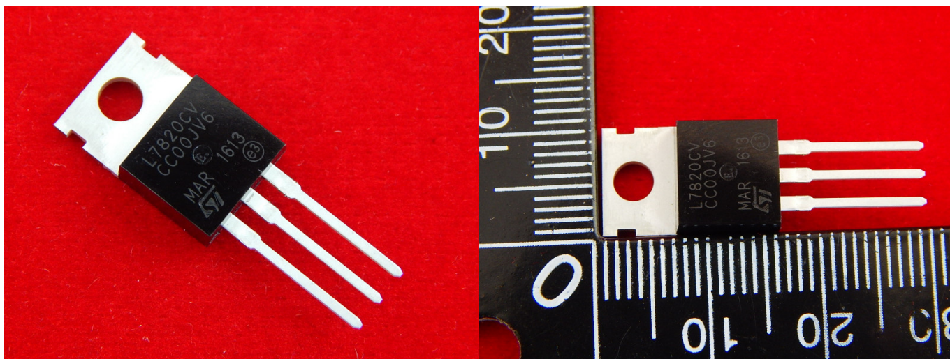
L7820CV Линейный стабилизатор 20В 1,0А Положительный
