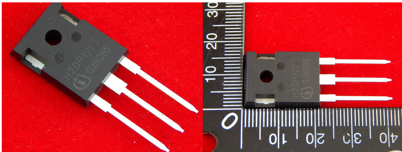
H20R1203, Транзистор 1200V 40A 310W [TO247-3]
