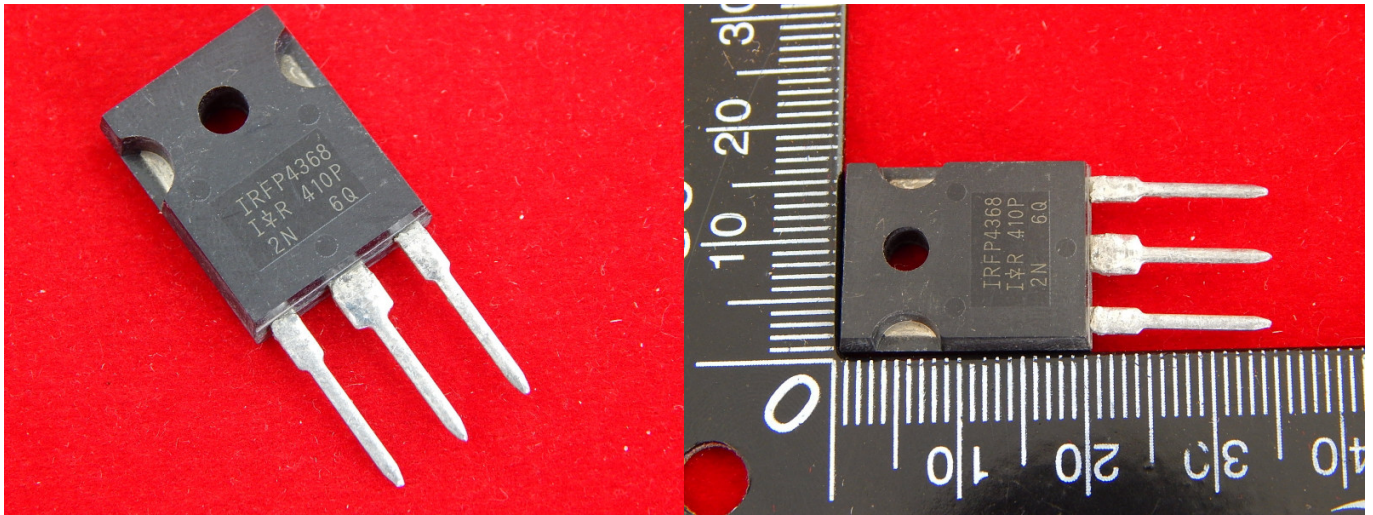
IRFP4368PBF, Транзистор, N-канал 75В 350А [TO-247AC]
