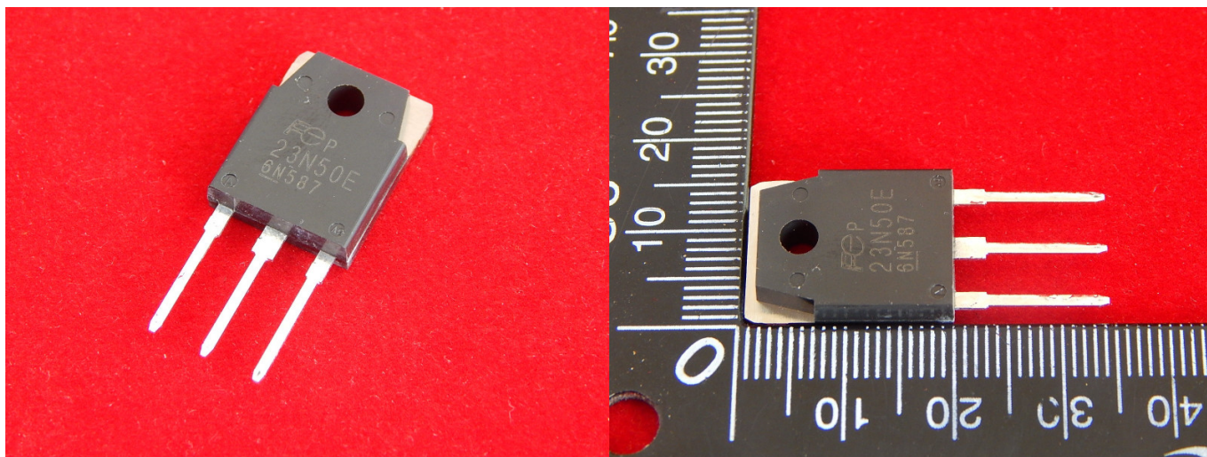
FMH23N50E, Транзистор, N-канал 500В 23А 0.245Ом [ТО-3P]
