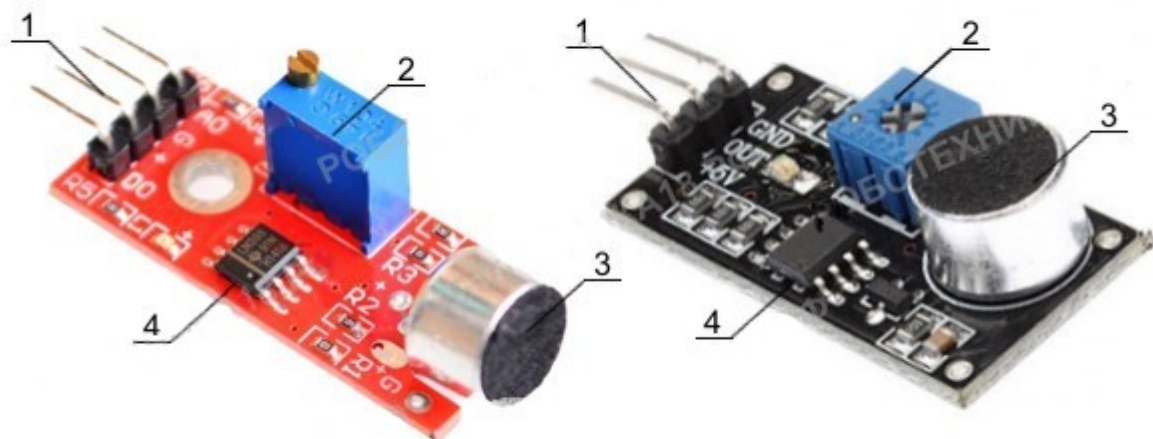
Устройство датчика звука
