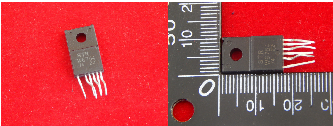
STRW6754, Импульсный регулятор напряжения [ТО-220-6]
