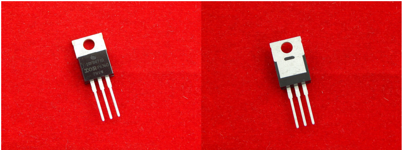
IRFB4710 Транзистор MOSFET, N-канал, 75 А, 100 V
