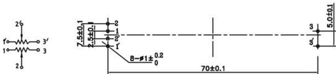
安装孔位图 Mounting Hole
