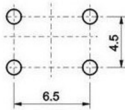
P.C.B.Land Pattern
