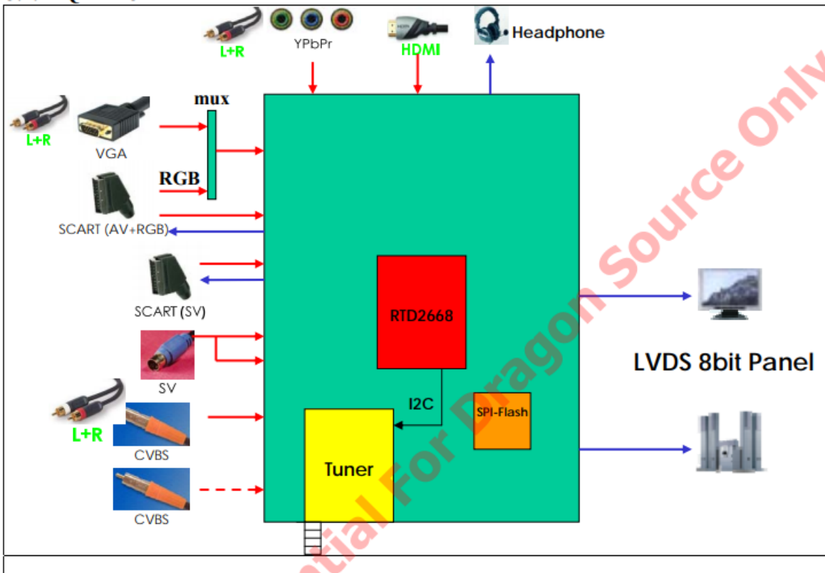
Схема подключения:
