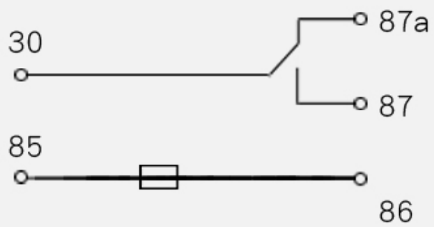
Пяти контактное реле
