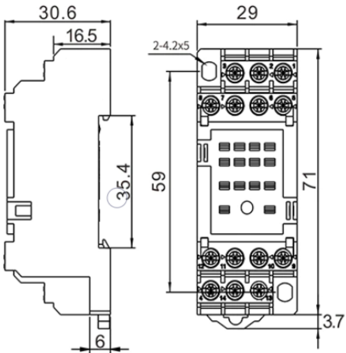
Габариты:
