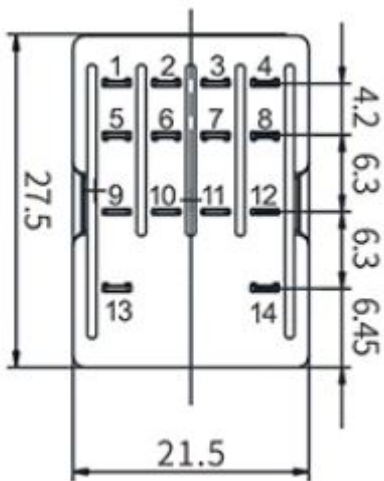
Габариты реле:
