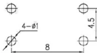
印制线路板 Recommended P.C.B layout
