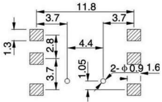
P.C.B. схема
